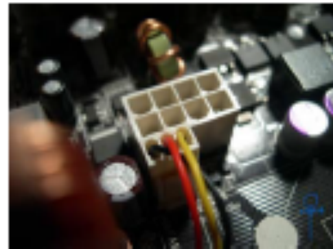
Conector hembra ATX P2 de 8 pines
