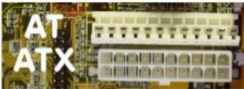
Conector hembra ATX P1 de 20 pines
