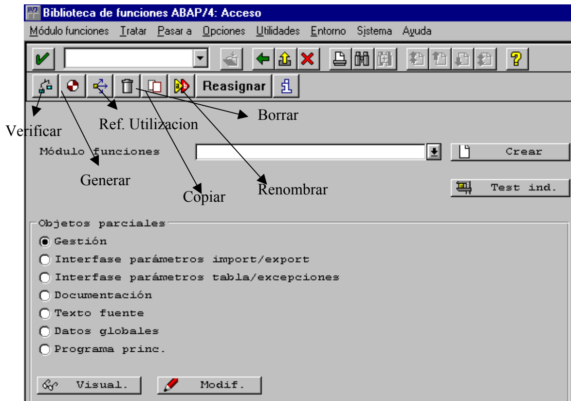
Fig. Biblioteca de funciones.
