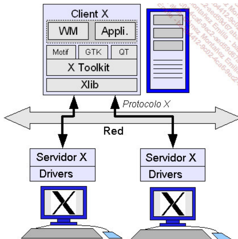
Arquitectura X Window
