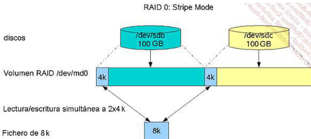
Fundamentos de RAID 0: Striping
