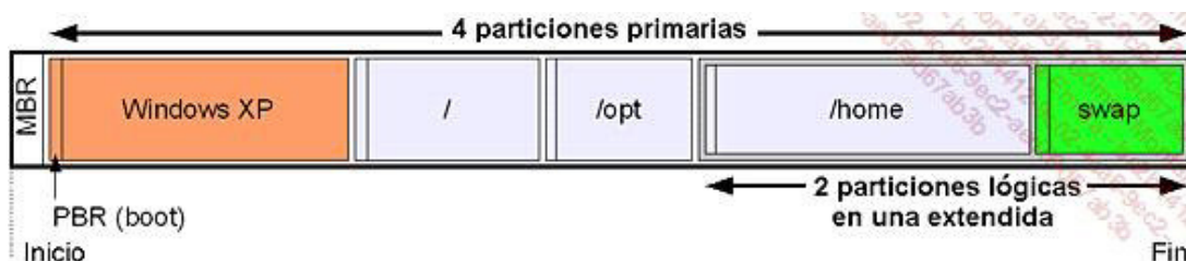
Descripción esquemática de un disco
