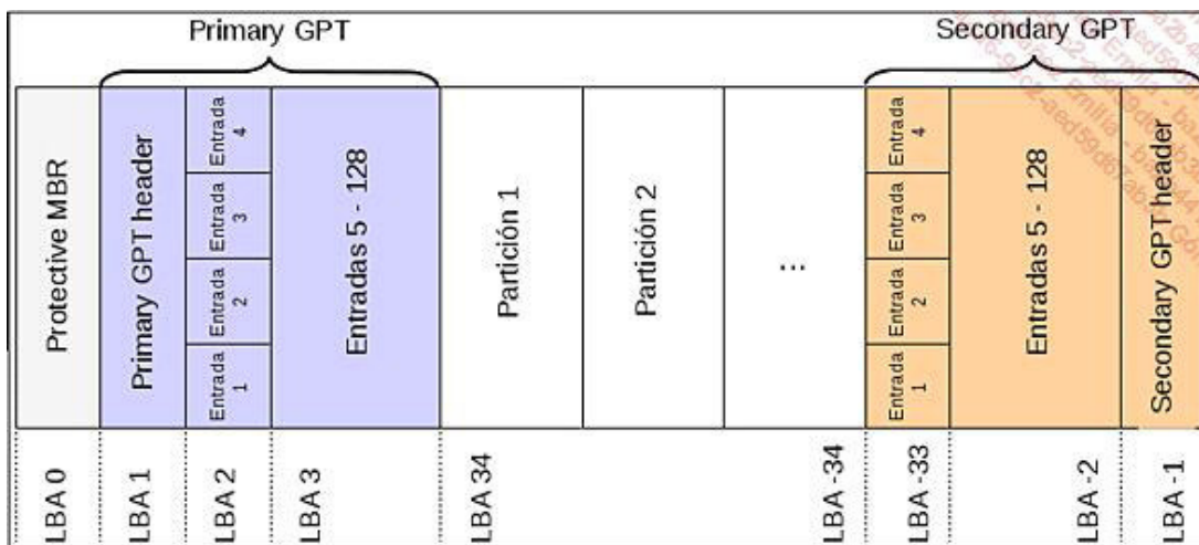
Estructura de un disco GPT
