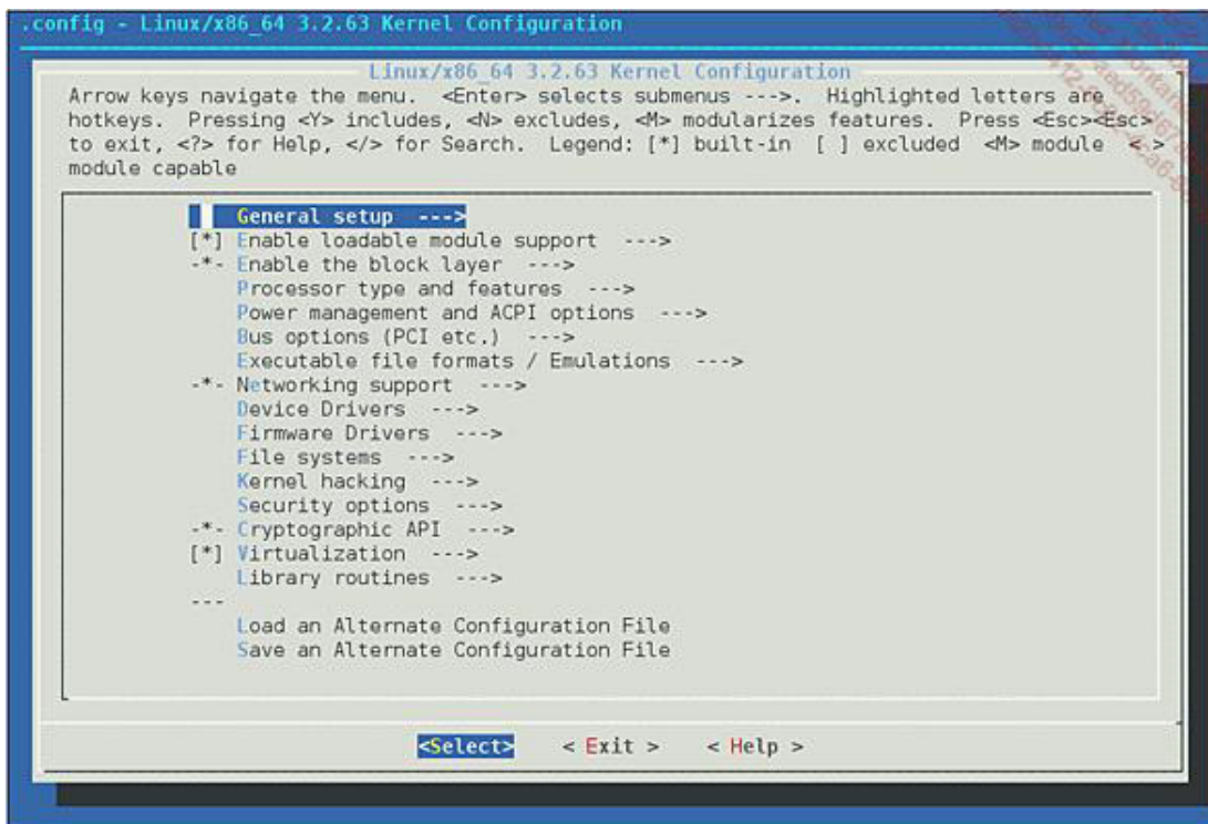
Las opciones de compilación del núcleo empleando menuconfig
