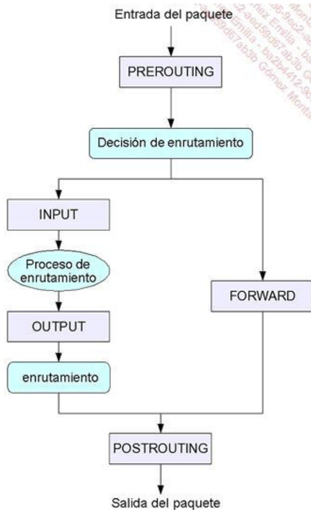
Las etapas de la vida de un paquete de red con netfilter
